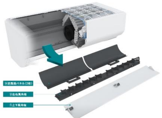
▲奥にある送風路まで取り外しが可能
